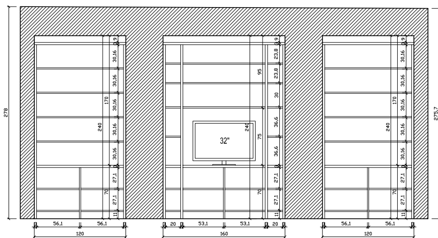
PRZEKRÓJ A-A
